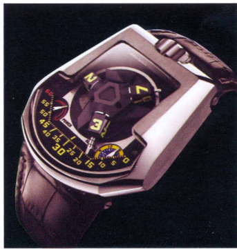
UR-201 45.6x15mm铂金与部份黑色钛合金表壳 / 回转立体卫星式时分指示，日夜及动力储存显示，仪表板可显示手动微调机制、保养警示及百年显示 / UR7.01手上链机芯 / 科技ARCAP P40材质面盘，钻石打磨卫星结构，超强夜光时分数字标示
